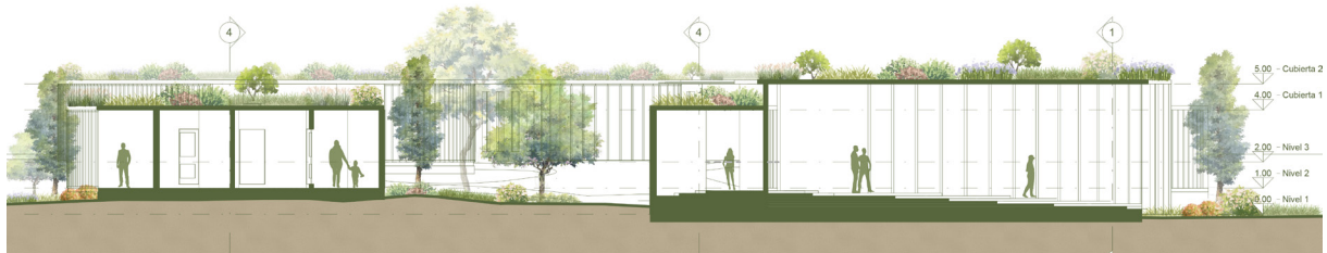
Figura 04 ▼ Corte general del proyecto.
